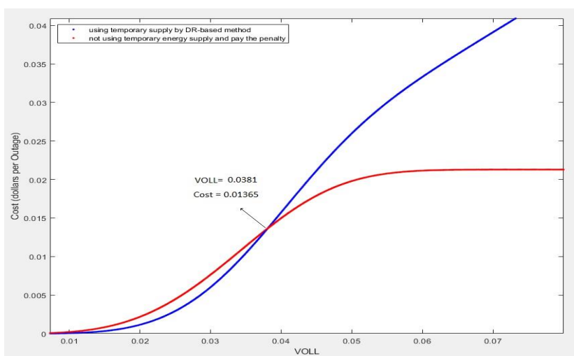
شکل ۱۰. نمودار تغييرات هزينه استفاده و عدم استفاده از روش تأمين موقت انرژي بر اساس مديريت تقاضا (با در نظر گرفتن تحليل حساسيت عرضه انرژي به قيمت پيشنهادي)
