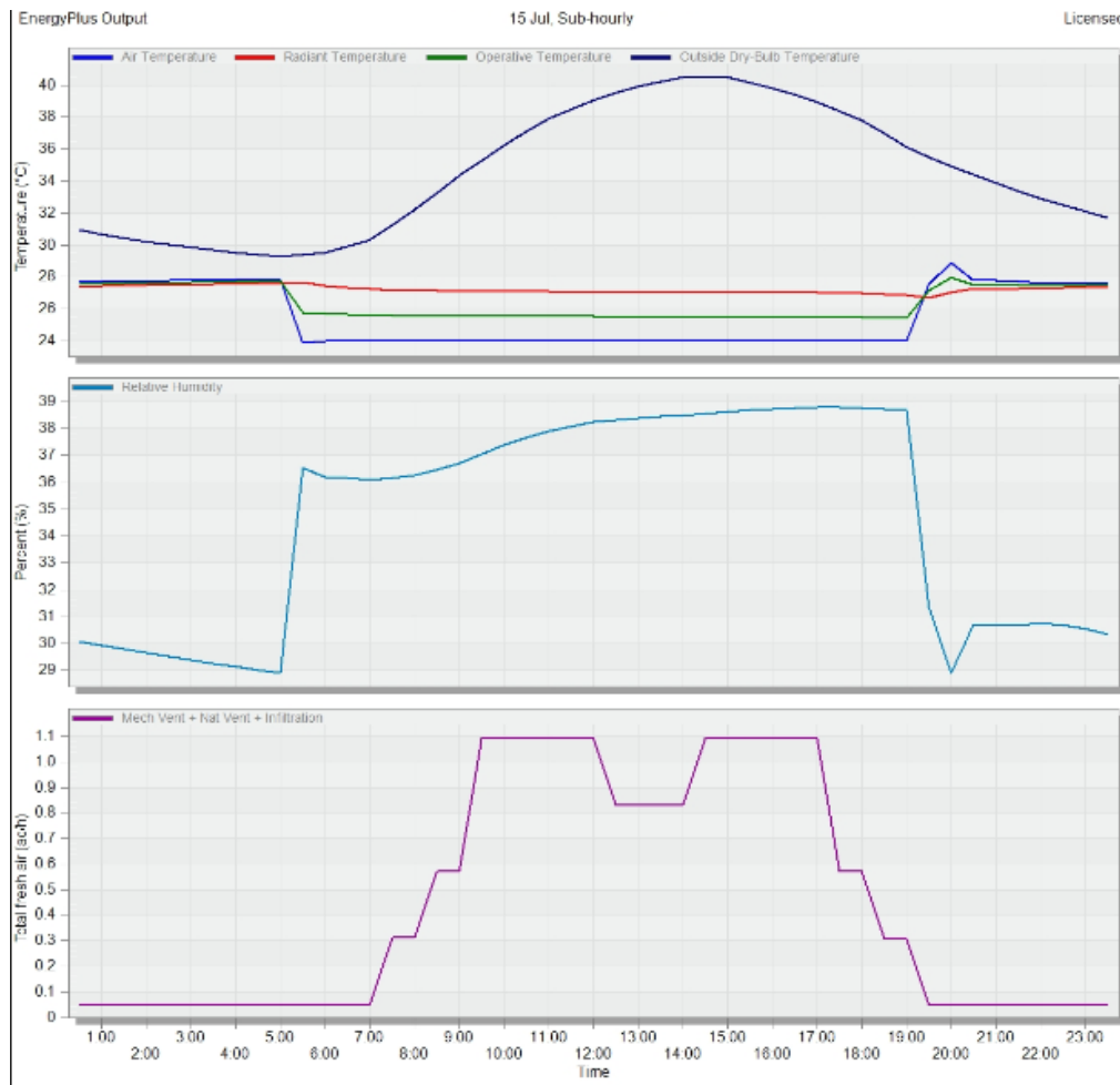
شکل ۱۰. دما، رطوبت نسبی و میزان هوای تازه ورودی به ساختمان
