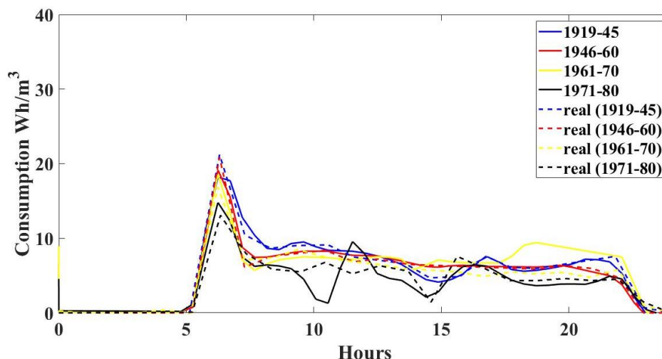
شکل ۱۱. نمودار مصرف انرژی با T_{ae}=12.5
