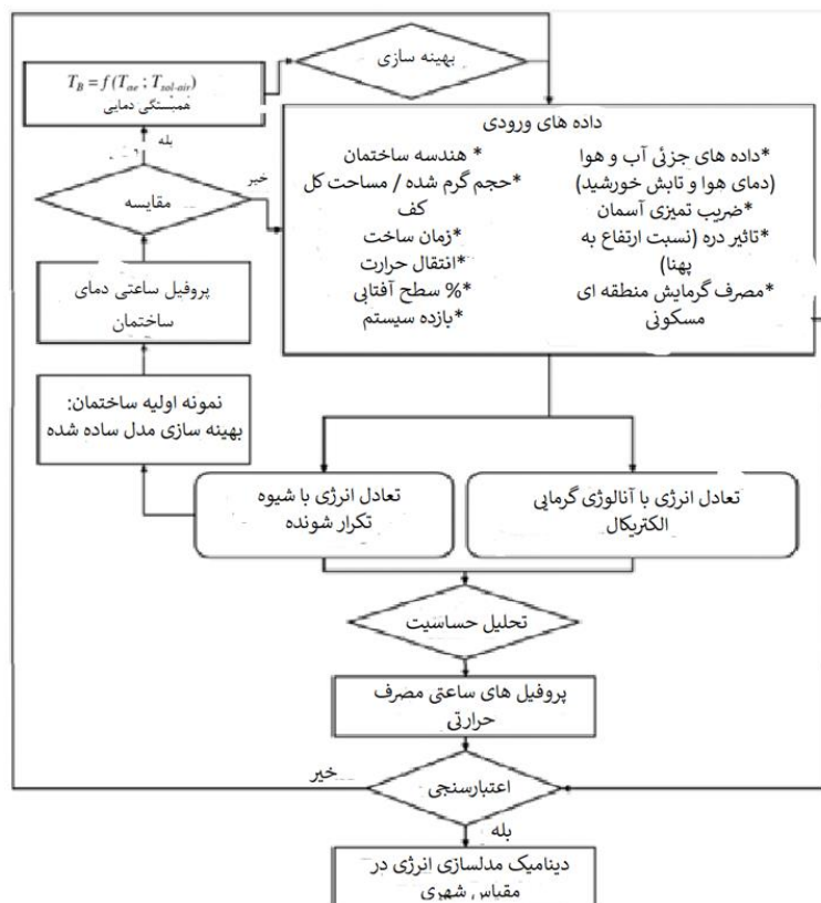
شکل ۱. فلوچارت روش کار
