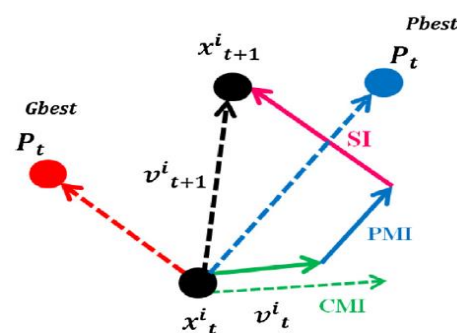
شکل ۲. به‌روزرسانی سرعت و موقعیت در الگوریتم بهینه‌سازی ازدحام ذرات
