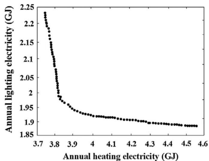
شکل ۸. بهینه‌سازی دوهدفه گرمایش- روشنایی در تهران
